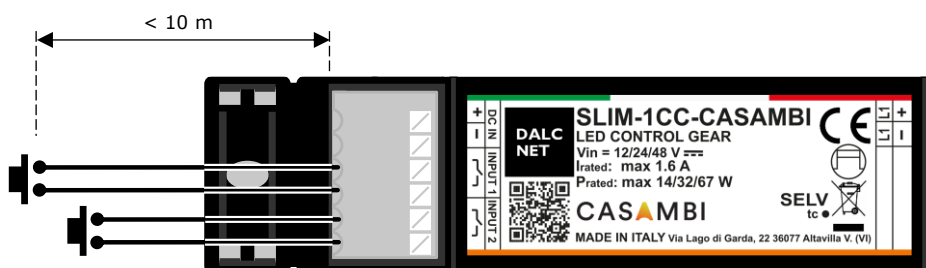
Figura 3: Schema di collegamento del comando locale per brevi distanze
