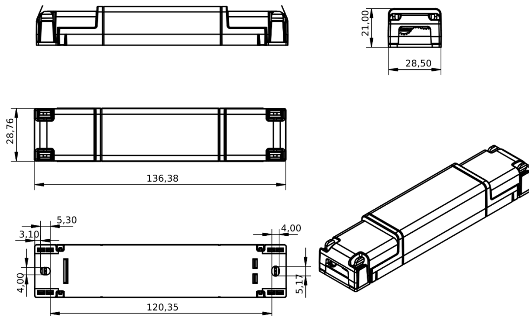
Figura 9: Dimensioni meccaniche
